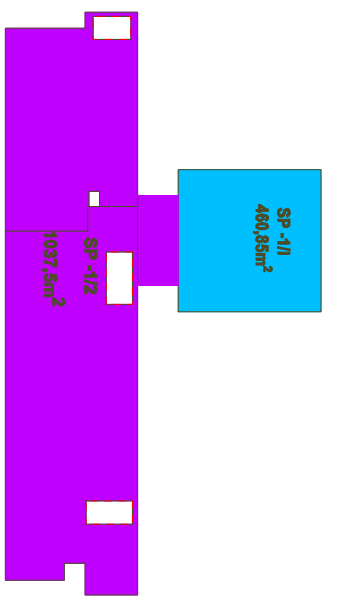
POZIOM 0 SCHEMAT PODZIAŁU NA STREFY P-POŻ.
